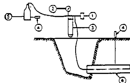
Διάταξη μέτρησης
