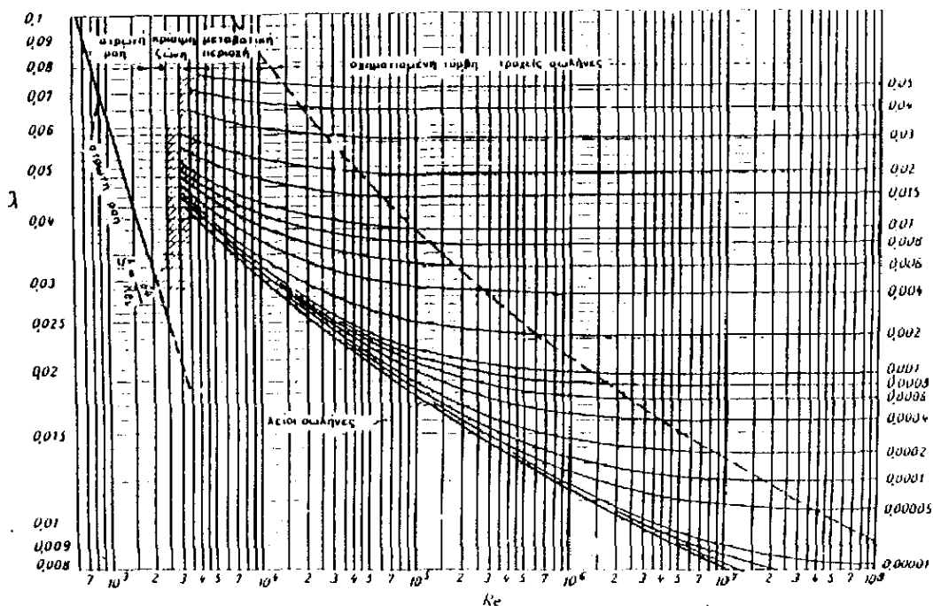
Διάγραμμα Moody: Συντελεστής αντίστασης \lambda για ροή σε σωλήνες
