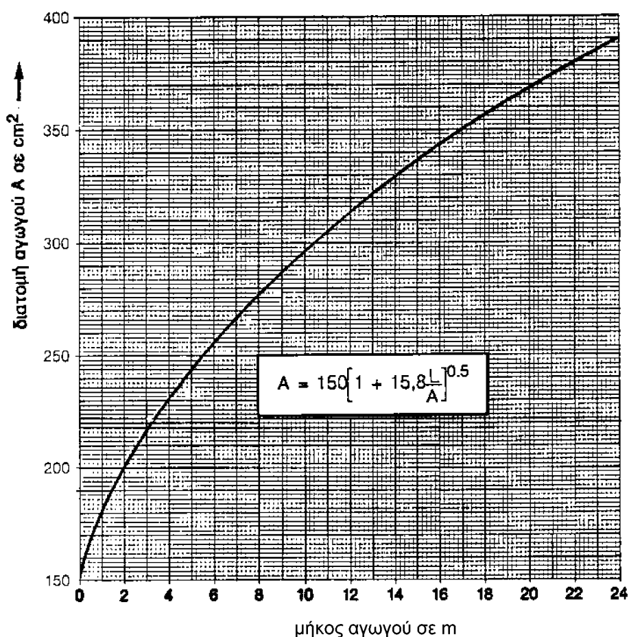
Διάγραμμα 8.1 Ισοδύναμη τετράγωνη διατομή αγωγού για αγωγό ελεύθερης διατομής 150 cm 2 εξαρτώμενη από το μήκος του αγωγού L
