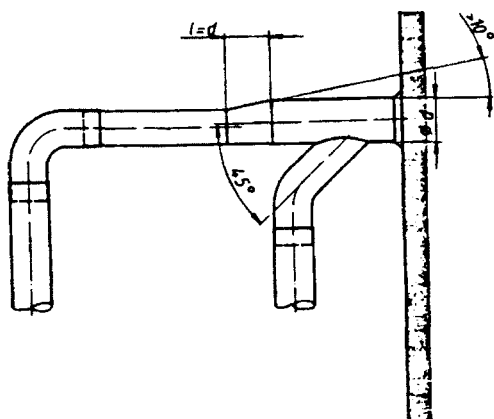
Εικόνα 9.1 Σχεδιασμός κοινού καπναγωγού
