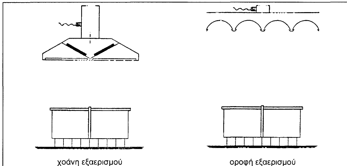
Εικόνα 13.1 Απαγωγή καυσαερίων συσκευών αερίου τύπου Α μέσω εγκαταστάσεων απορροφητήρων
