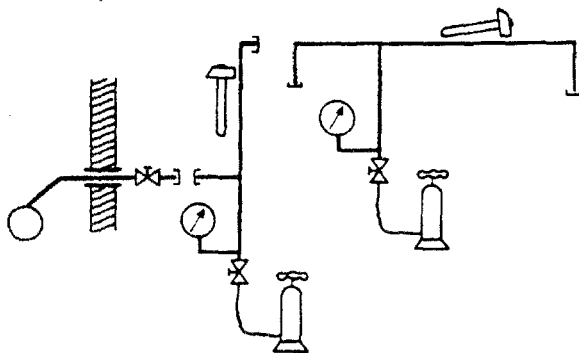
Εικόνα 10.1 Δοκιμή αντοχής
