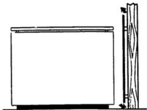
Εικόνα 10.1 Παράδειγμα για αεριζόμενη προστασία έναντι θερμικής ακτινοβολίας
