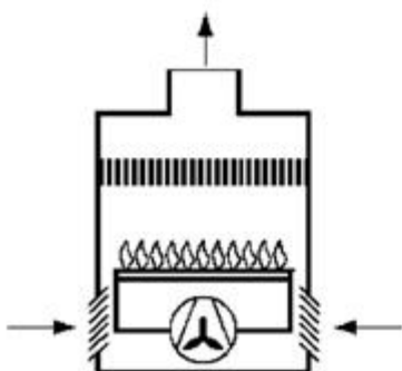
B 23 με ανεμιστήρα πριν τον καυστήρα
