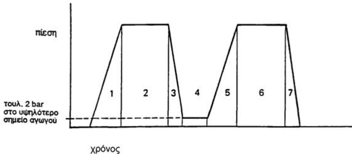
Εικ. 12.3 Χρονική πορεία μιας δοκιμής πίεσης
