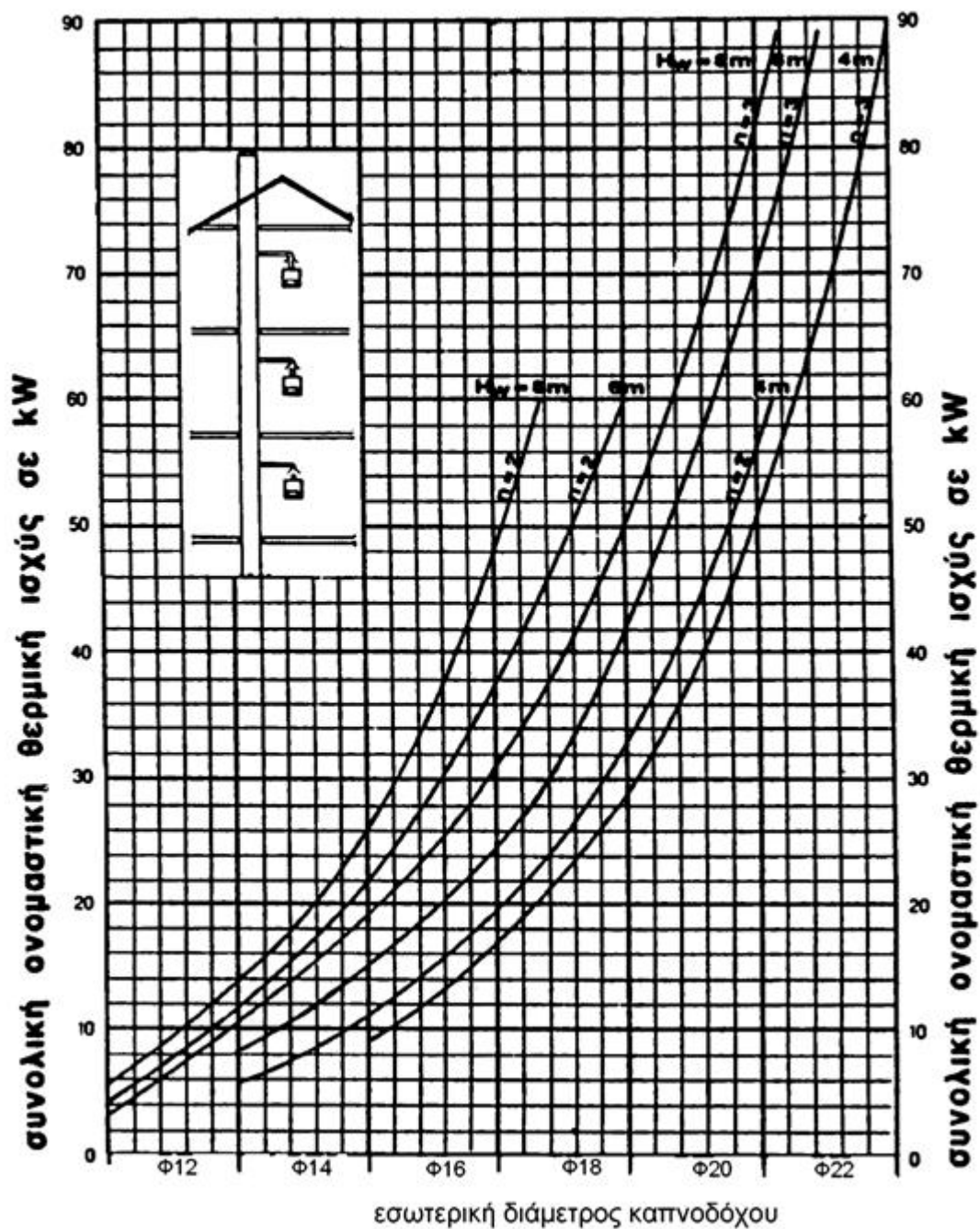
Εικ. 6 Κοινή καπνοδόχος για συσκευές χωρίς ανεμιστήρα
