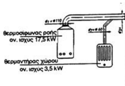
Εικόνα 11.2 Σύνδεση με κοινό καπναγωγό θερμαντήρα νερού και θερμαντήρα χώρου
