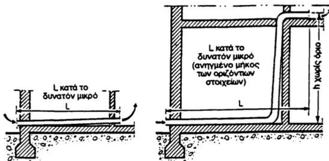
Εικόνα 10.4 Παραδείγματα οδήγησης αγωγών τροφοδοσίας αέρα καύσης
