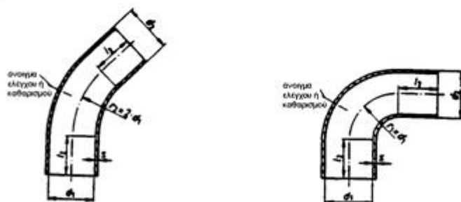
Εικ.11.6 Στοιχεία μορφής κατυναγωγών από μέταλλο
