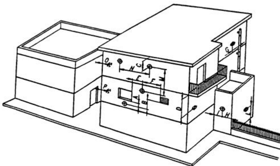
Εικόνα 10.8 Αποστάσεις στομίων συσκευών αερίου
