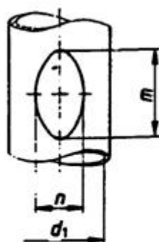
Εικ.11.7 Ανοίγματα καθαρισμού και ελέγχου κατυναγωγών από μέταλλο
