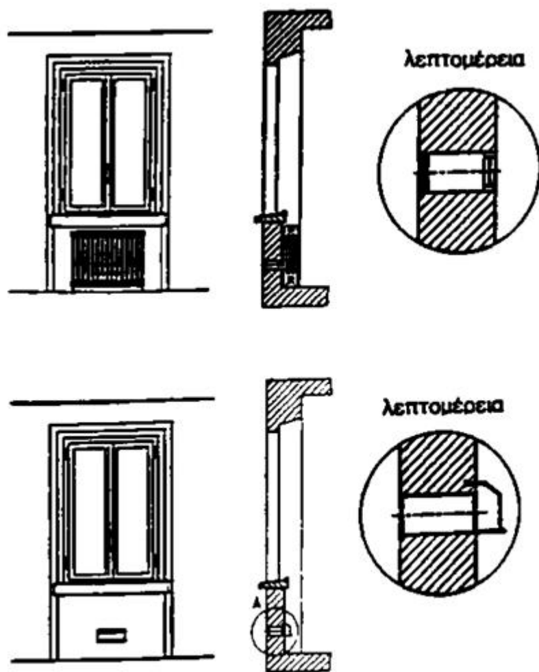
Εικόνα 10.3 Παραδείγματα θέσεων ανοιγμάτων τροφοδοσίας αέρα καύσης
