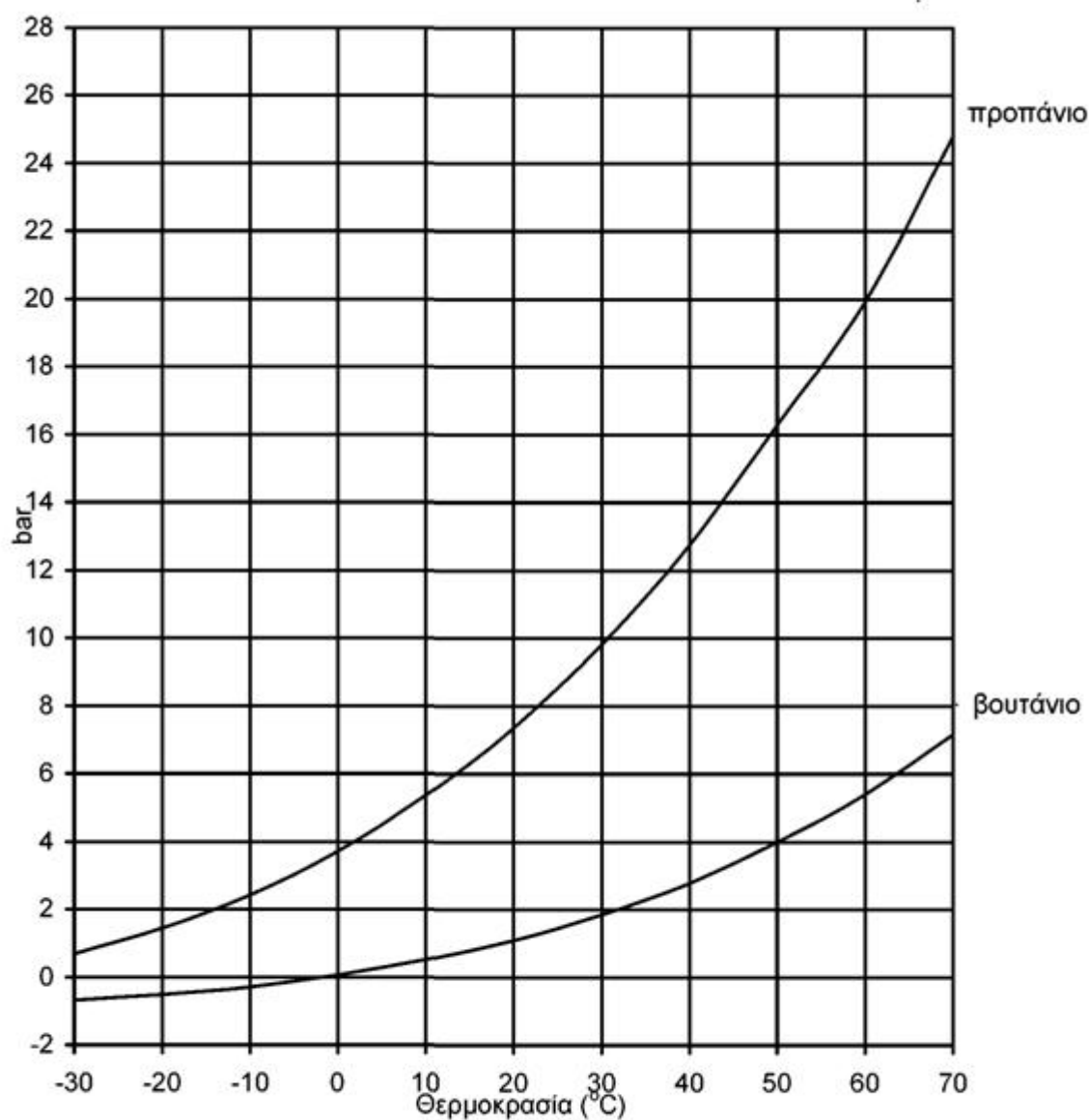
Εικ. 1 Καμπύλες (υπερ)πίεσης ατμών
