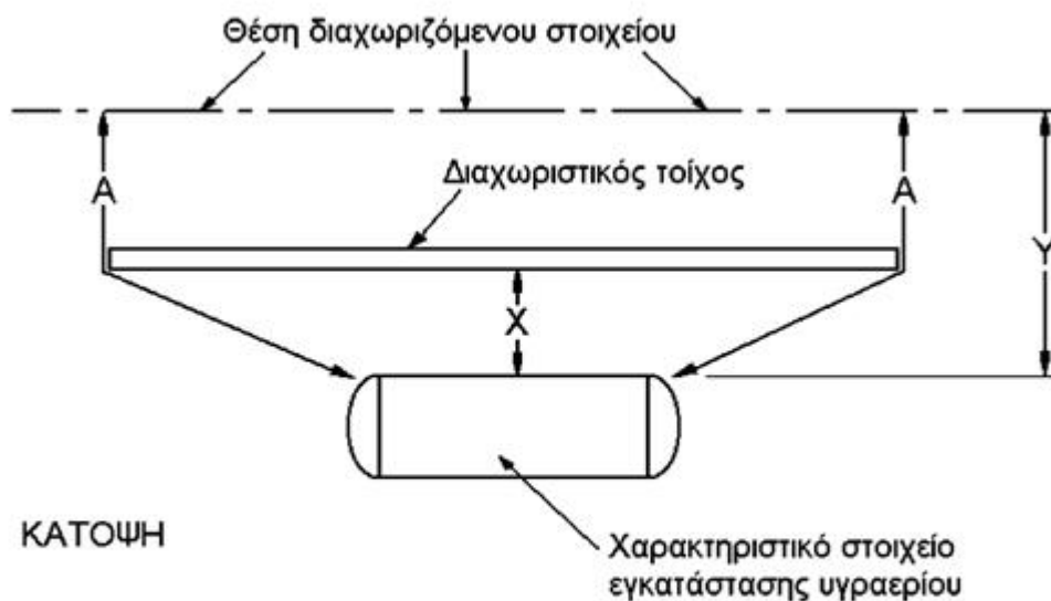
Εικόνα 5.1 Καθορισμός μήκους διαχωριστικού τοίχου
