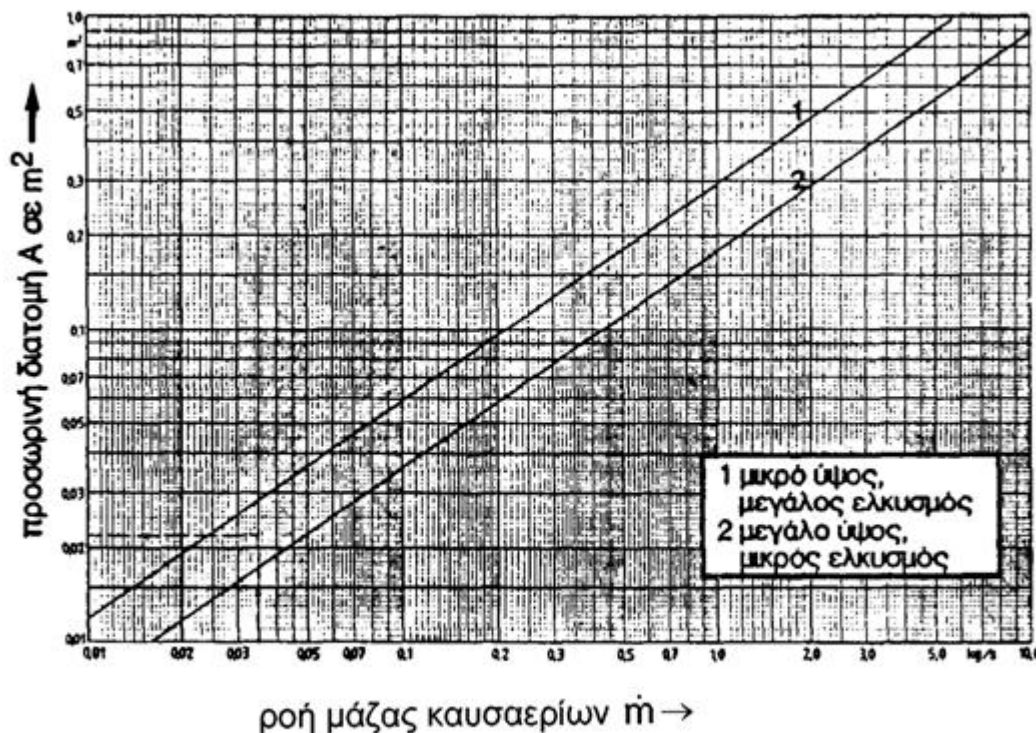
Εικόνα 2 Προεκτίμηση της διατομής της καπνοδόχου
