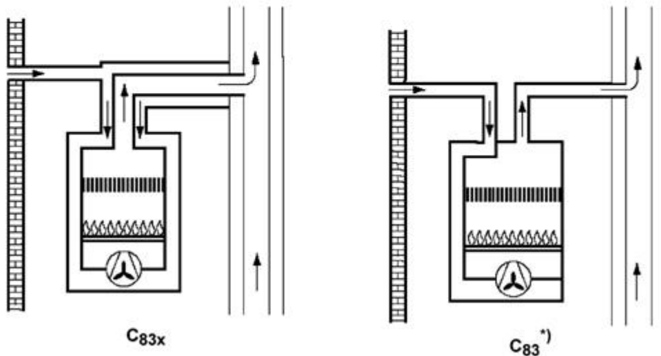
C83 με ανεμιστήρα πριν τον καυστήρα
