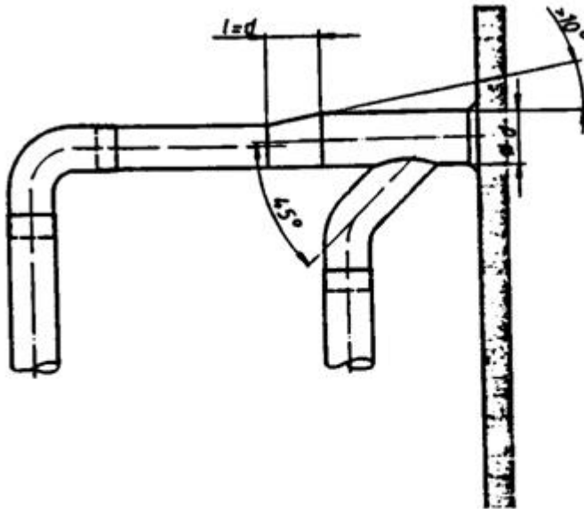
Εικόνα 11.1 Σχεδιασμός κοινού καπναγωγού
